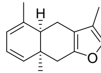
Tubipofuran
