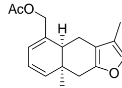
15-acetoxytubipofuran
