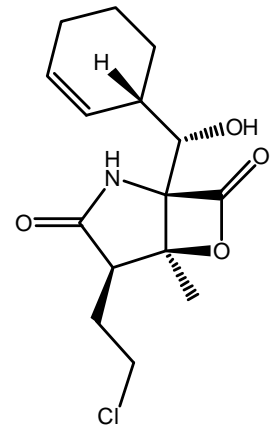
Salinosporamide A
